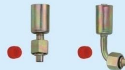
YM-1063 全铁接头 Iron adapter 3/8 O 180°
